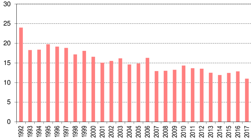
Stickstoffdioxid - Jahresmittelwerte
