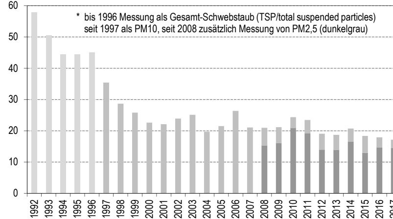
Partikel* - Jahresmittelwerte
