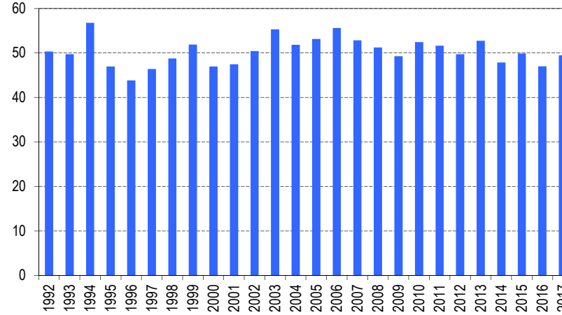
Ozon - Jahresmittelwerte
