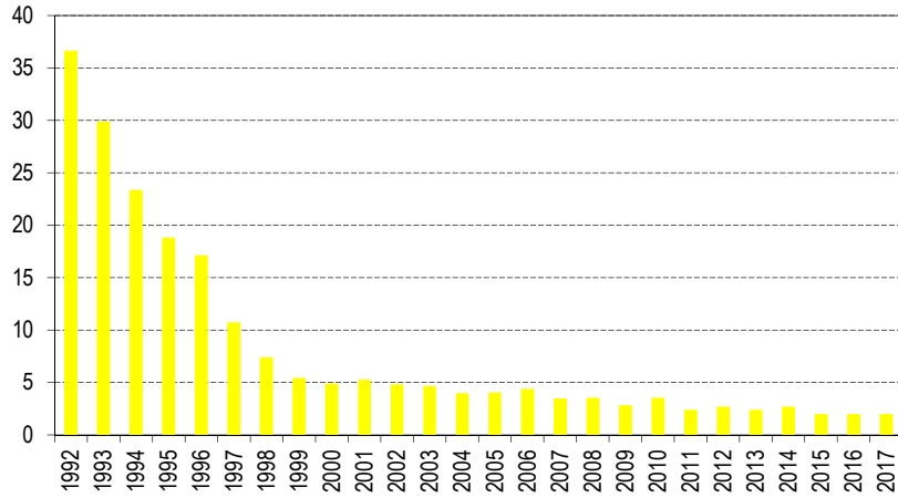
Schwefeldioxid - Jahresmittelwerte
