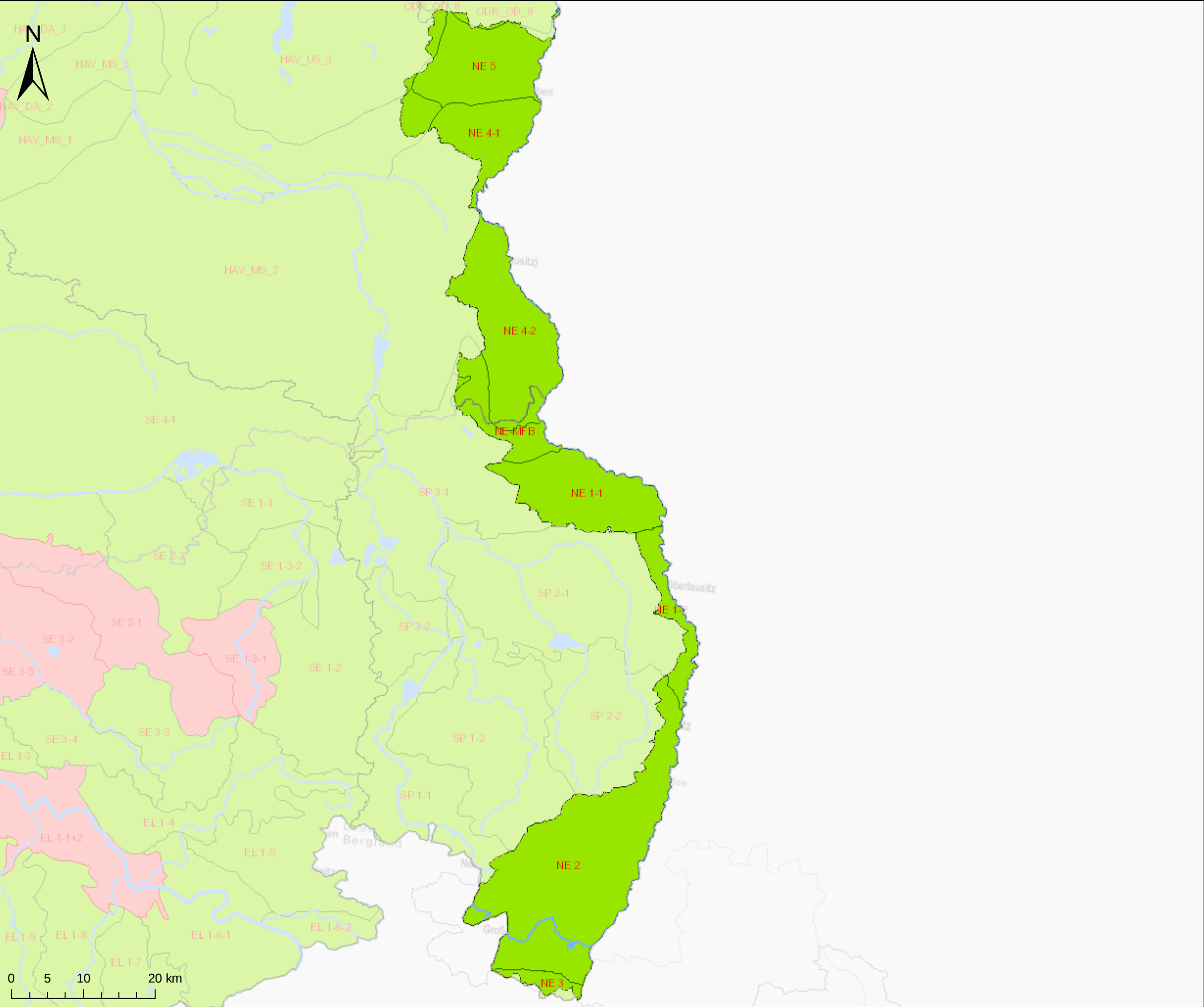
FGE Oder, BG LAN, Karte 4.6.1: Chemischer Zustand der Grundwasserkörper hinsichtlich Nitrat
