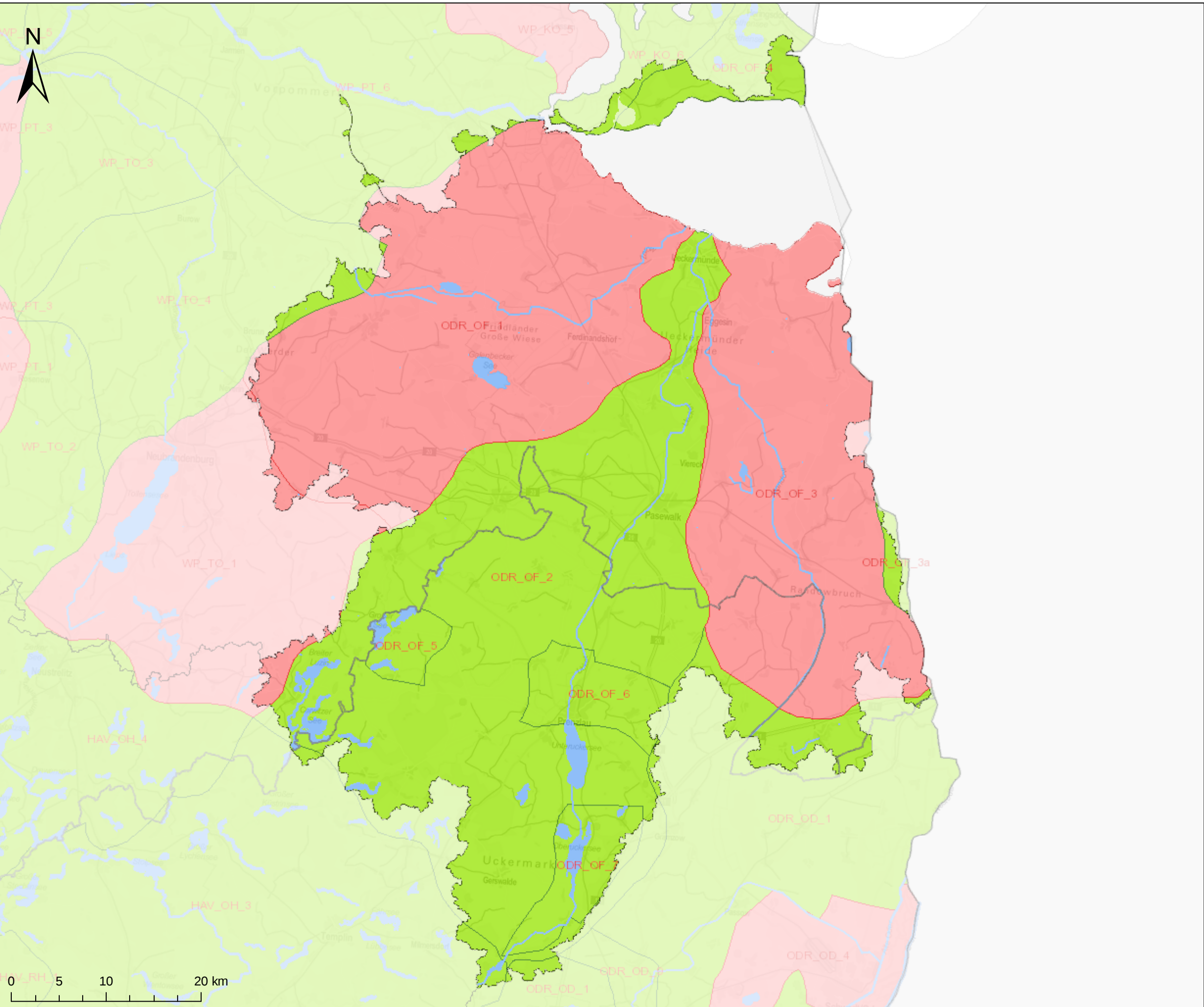
FGE Oder, BG Stettiner Haff, Karte 4.6: Chemischer Zustand der Grundwasserkörper und Identifikation von Grundwasserkörpern mit signifikant zunehmendem Schadstofftrend
